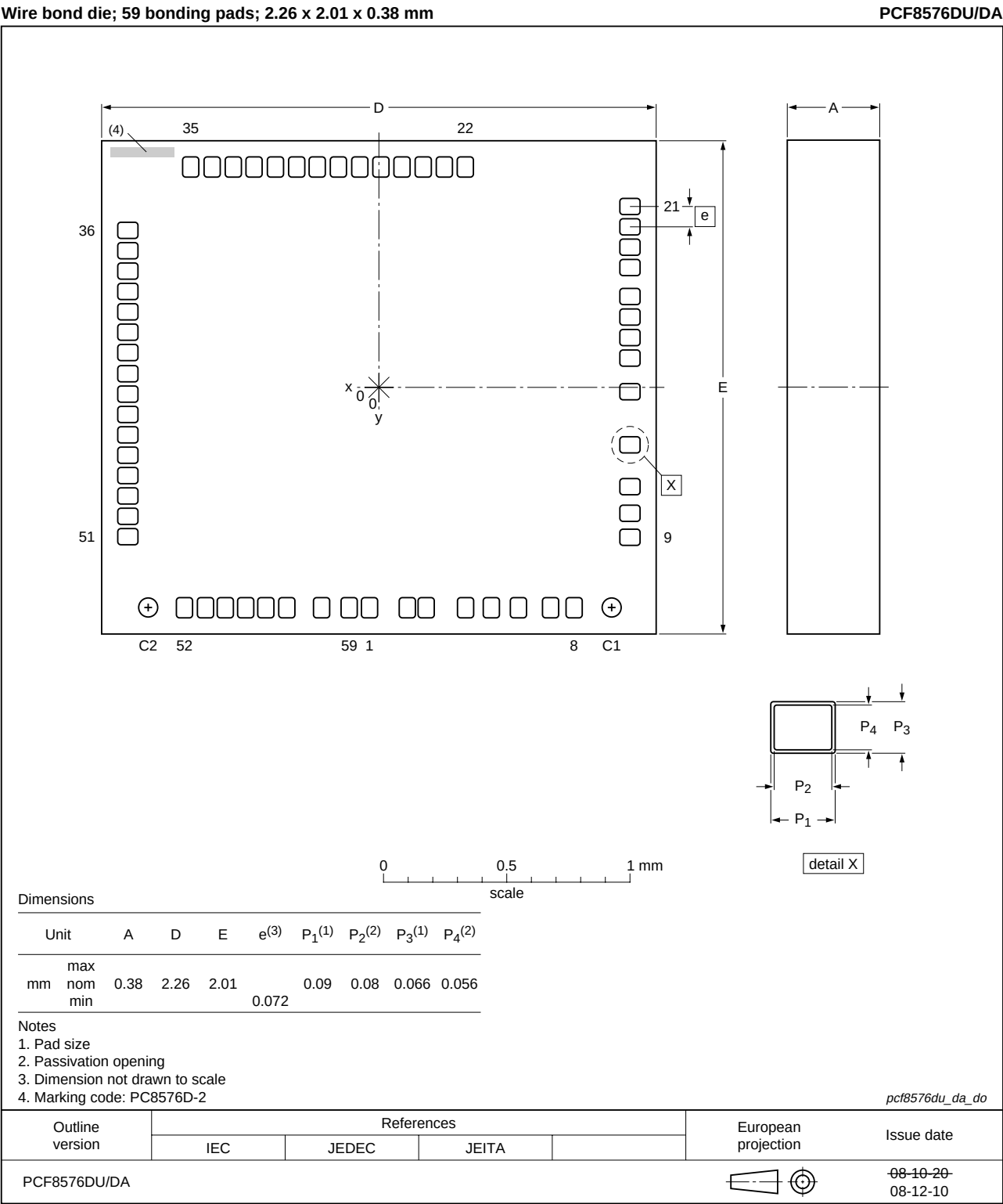
Fig 26. Bare die outline PCF8576DU/DA/2
